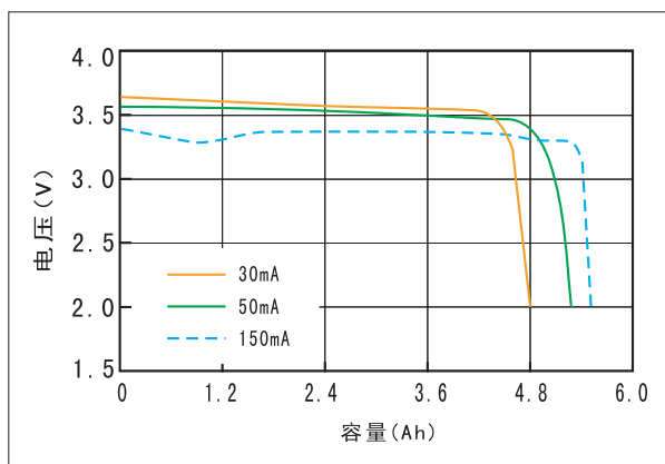
150℃放电曲线
