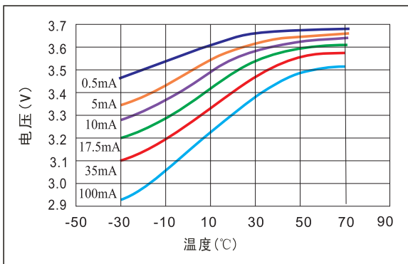
电压与温度关系曲线
