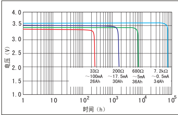
25°C放电特性
