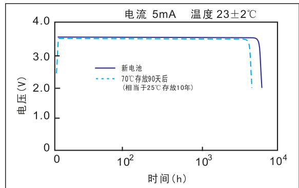
存储放电特性
