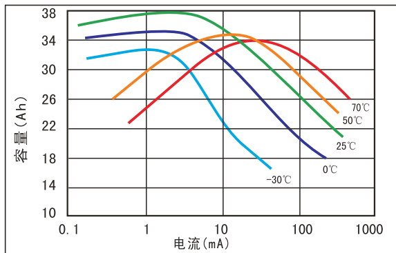
容量与电流关系曲线 (2.0V终止)
