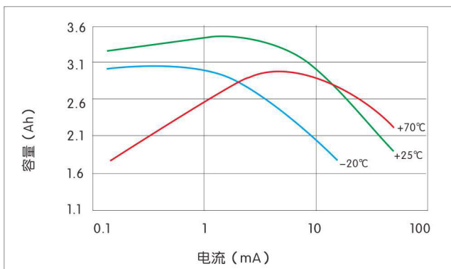
容量与电流关系曲线
