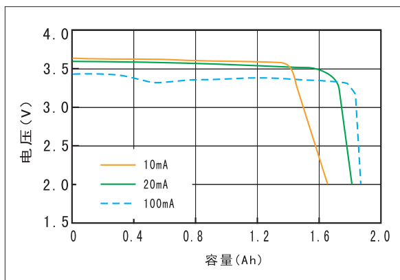
150℃放电曲线
