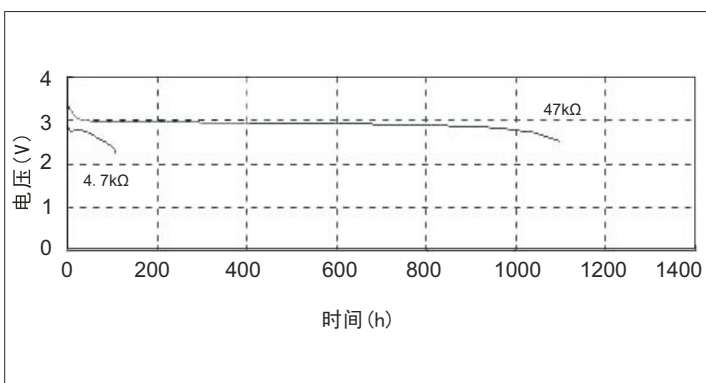
25℃放电曲线
