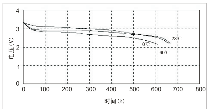
不同温度下放电曲线(62kΩ)
