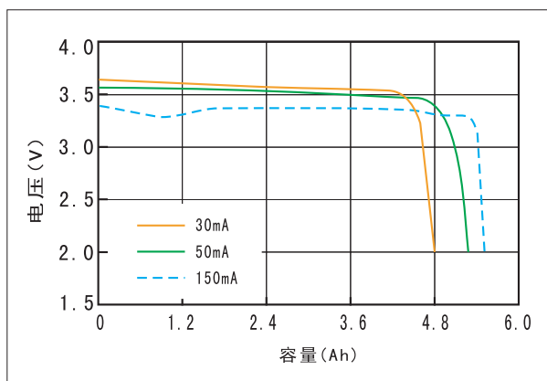
150℃放电曲线
