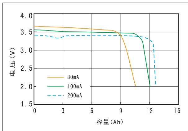
150℃放电曲线
