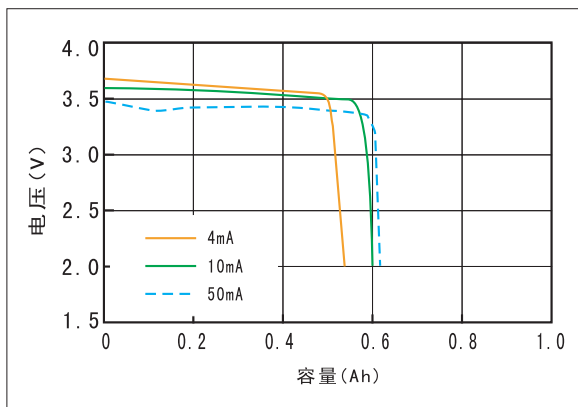
150°C 放电曲线
